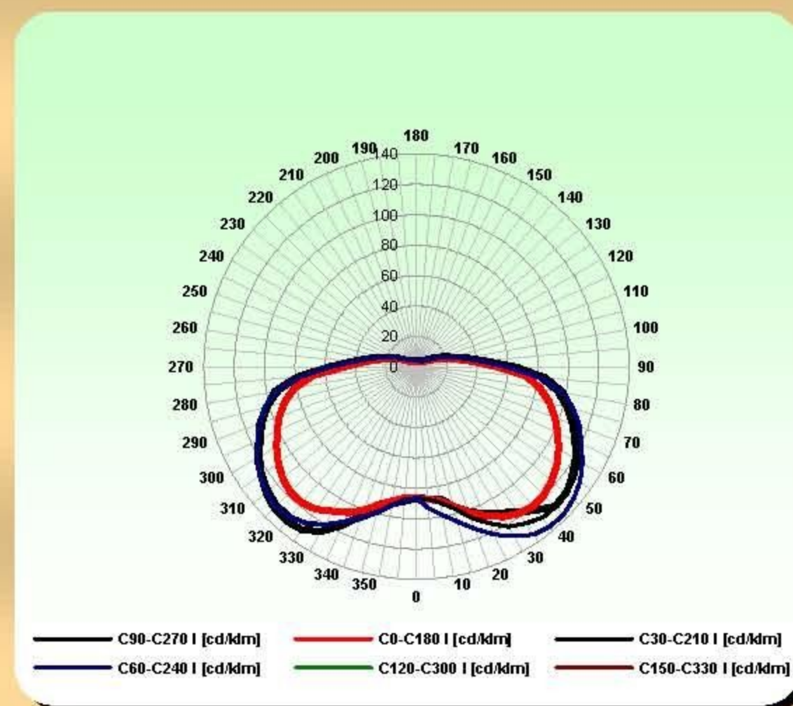
Fotometrická křivka
