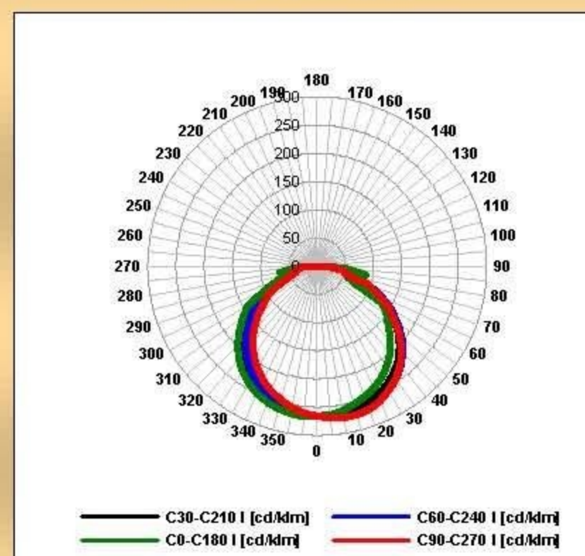
fotometrická křivka
